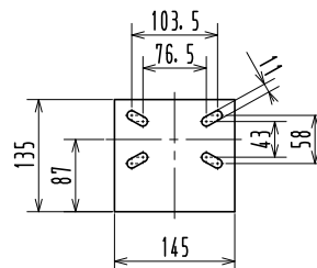
固定車用キャスト一板詳細
