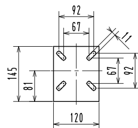
自在車用キャスト一板詳細
