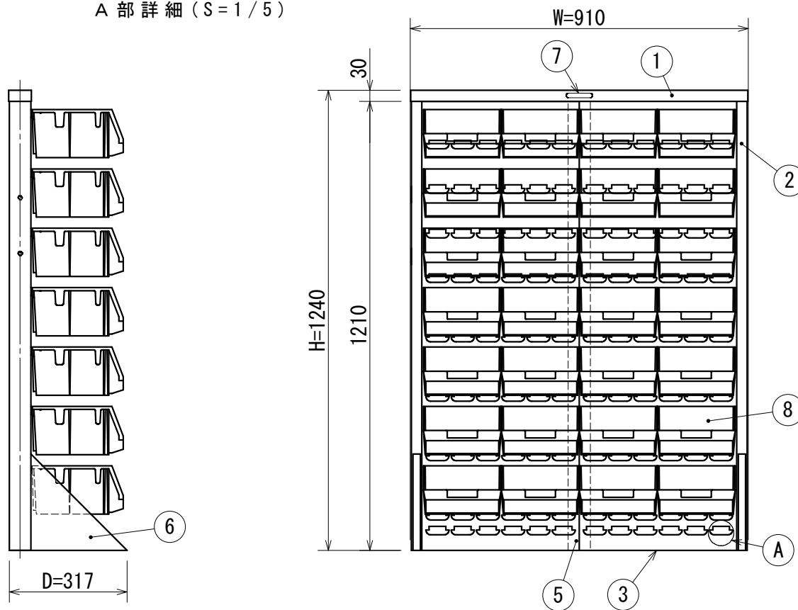
A 部 詳 細 ( S = 1 / 5 )
