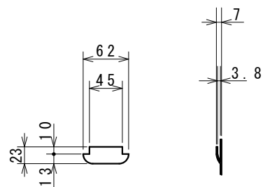
A 部 詳 細 ( S = 1 / 5 )
