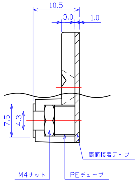
A-B断面図
