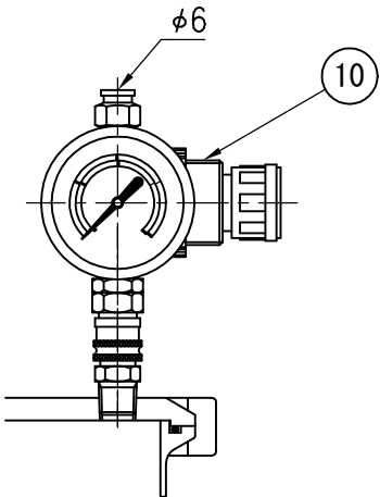
*A (バルブ詳細)
