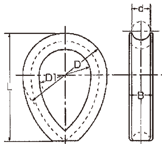
ワイヤロープ用 A型シンブル
