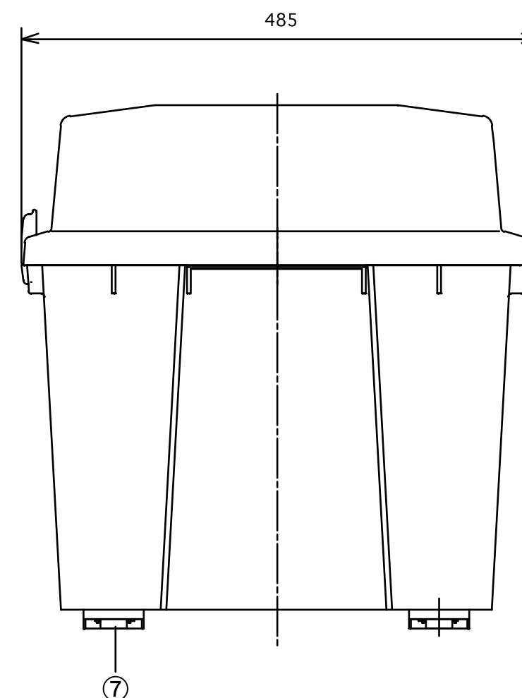
側面視
