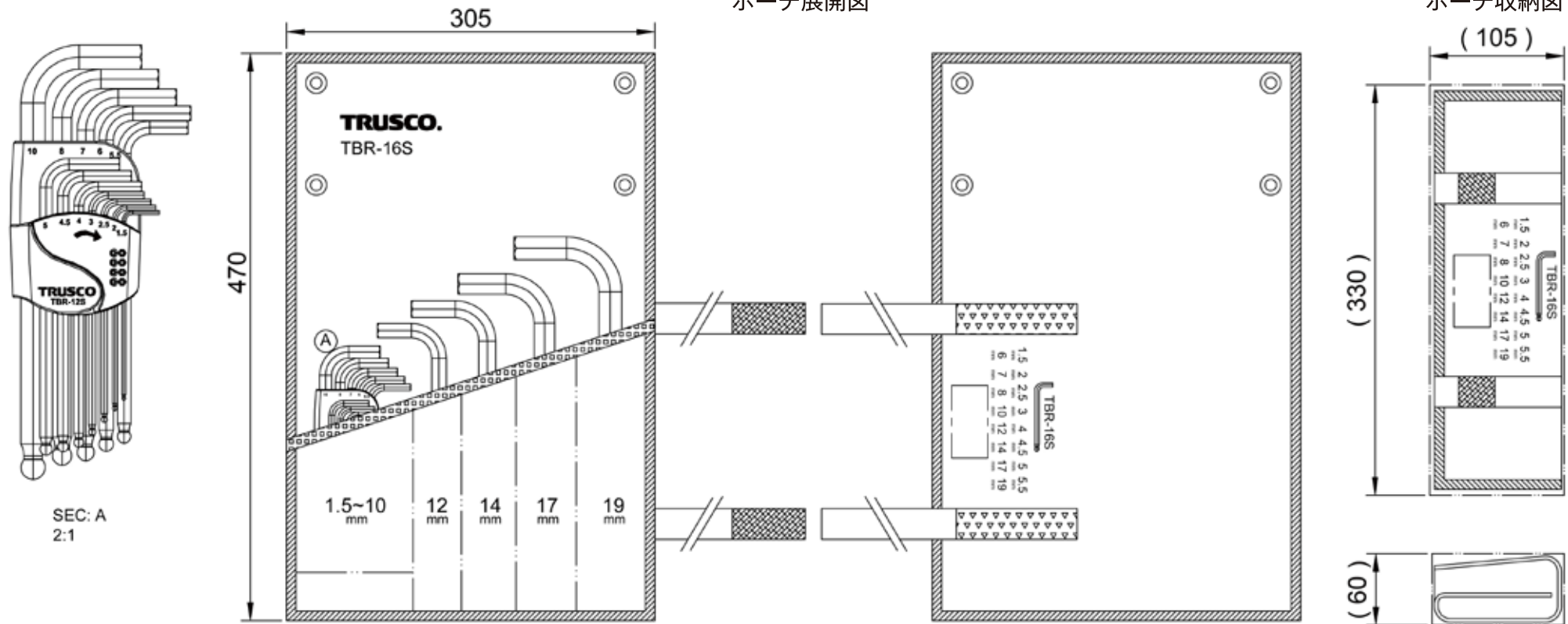
ポーチ展開図
