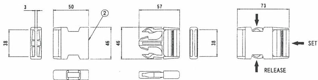
バックル詳細図
