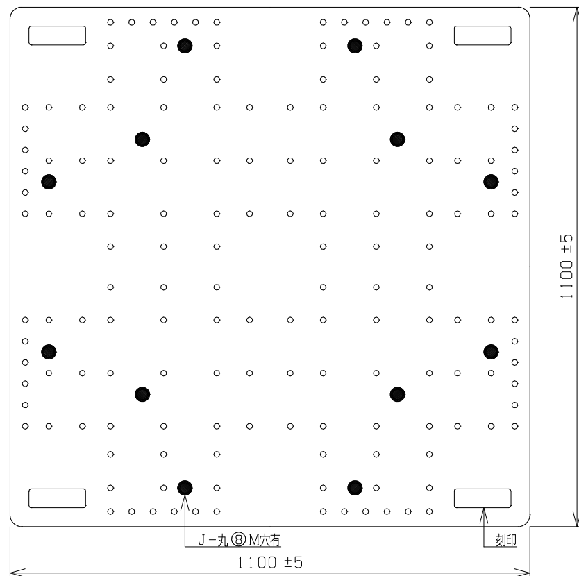
上面図
