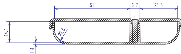
C-C断面図
