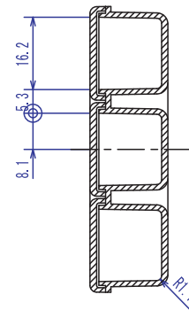
A-A断面図
