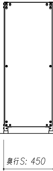
側面図
