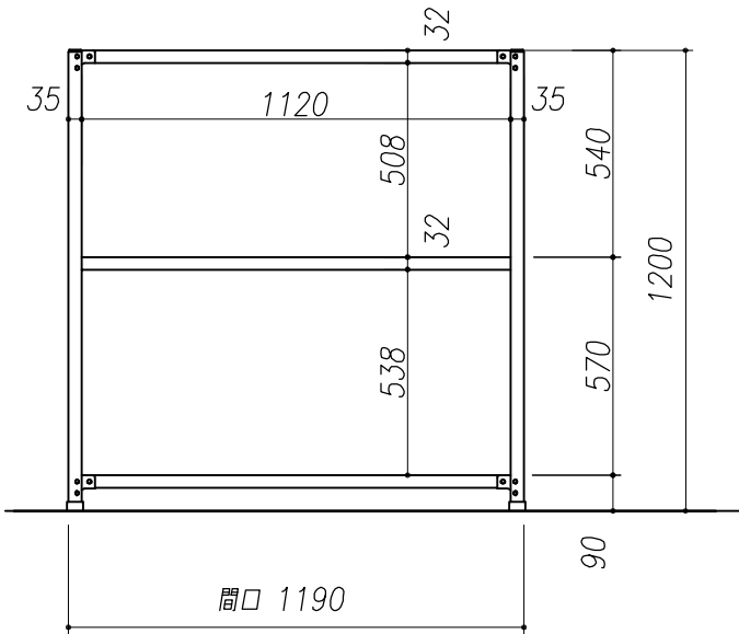
正面図
