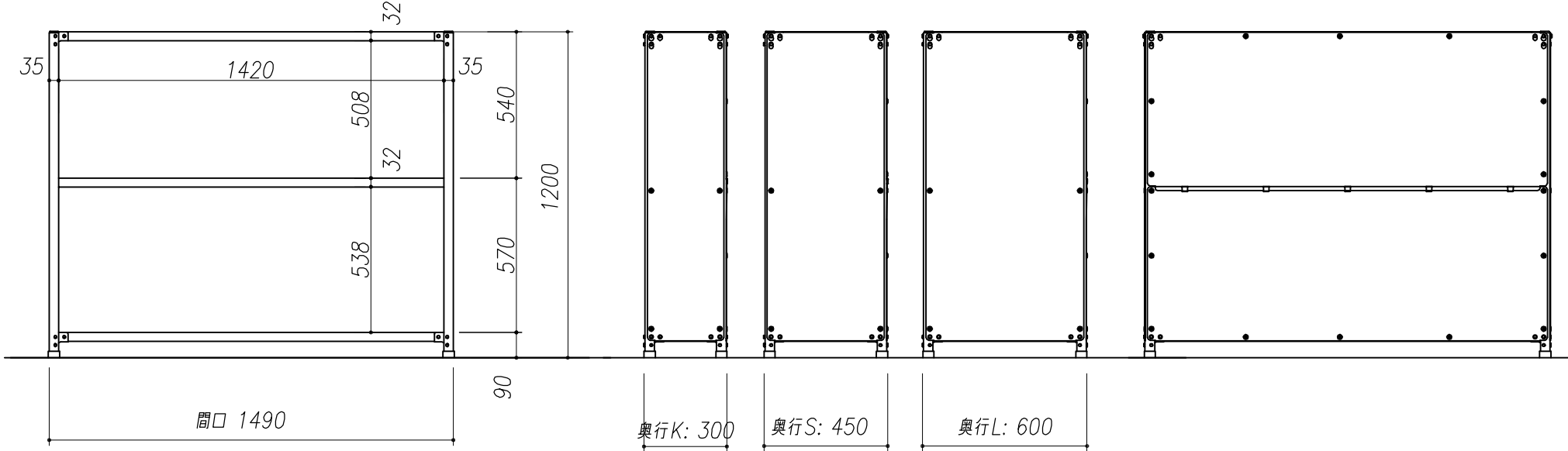
正面図
