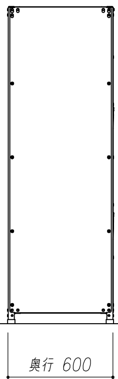
側面図
