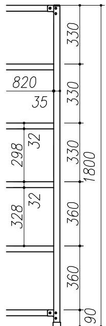
品番： TLA63S-26D
