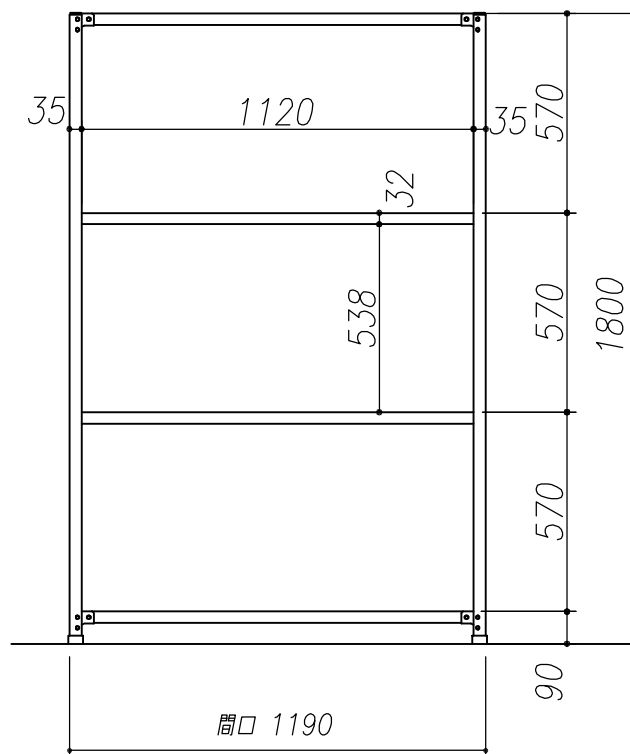
正面図
