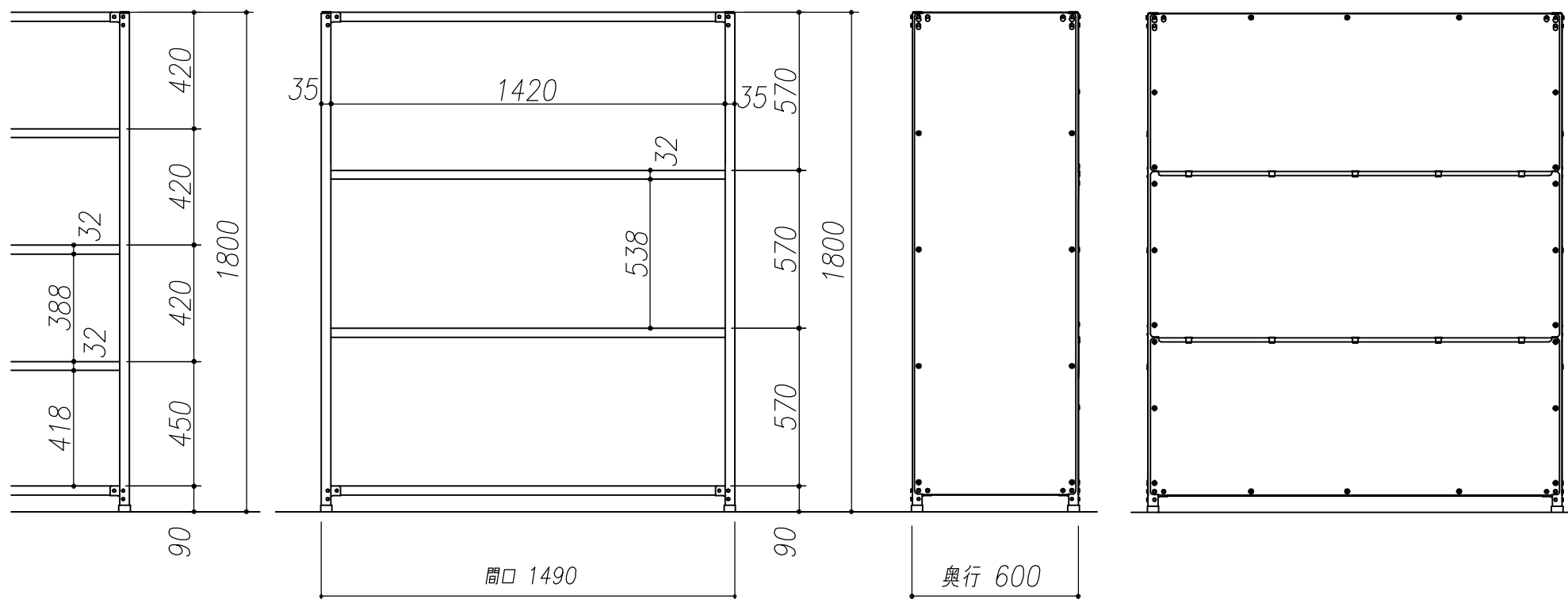
正面図
