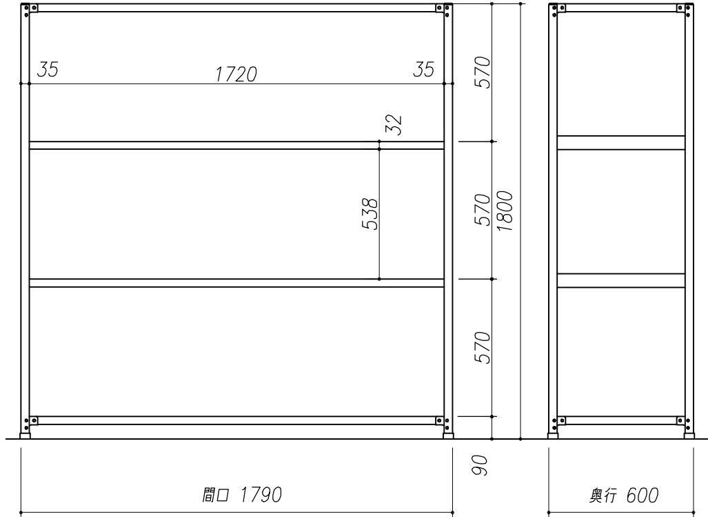
品番：TLA66L-14
