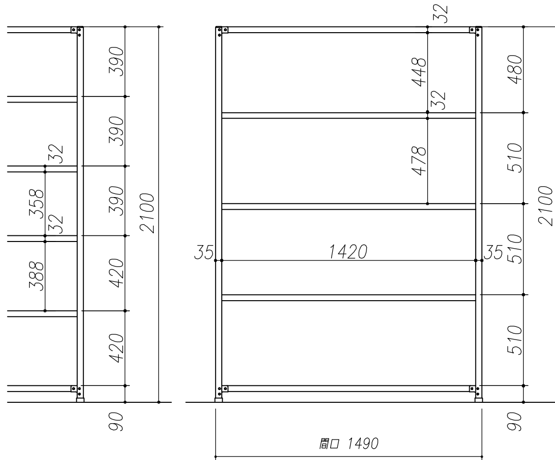
正面図
