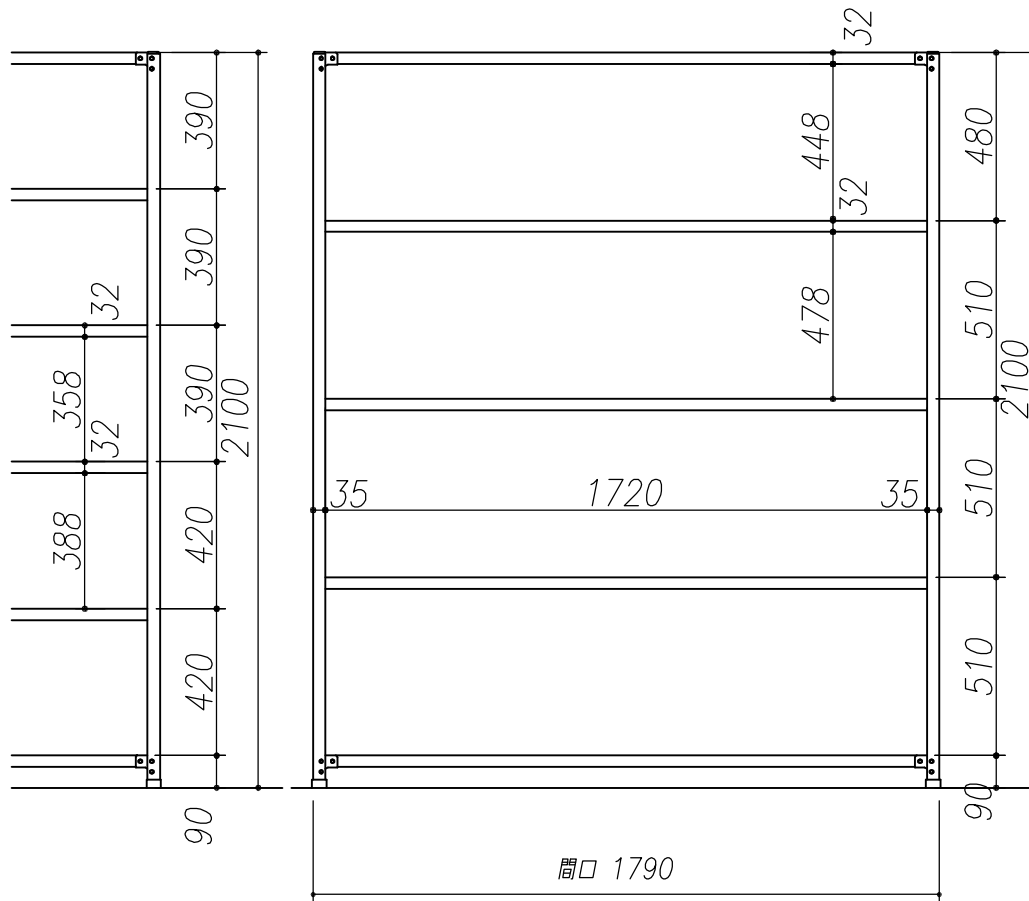
正面図
