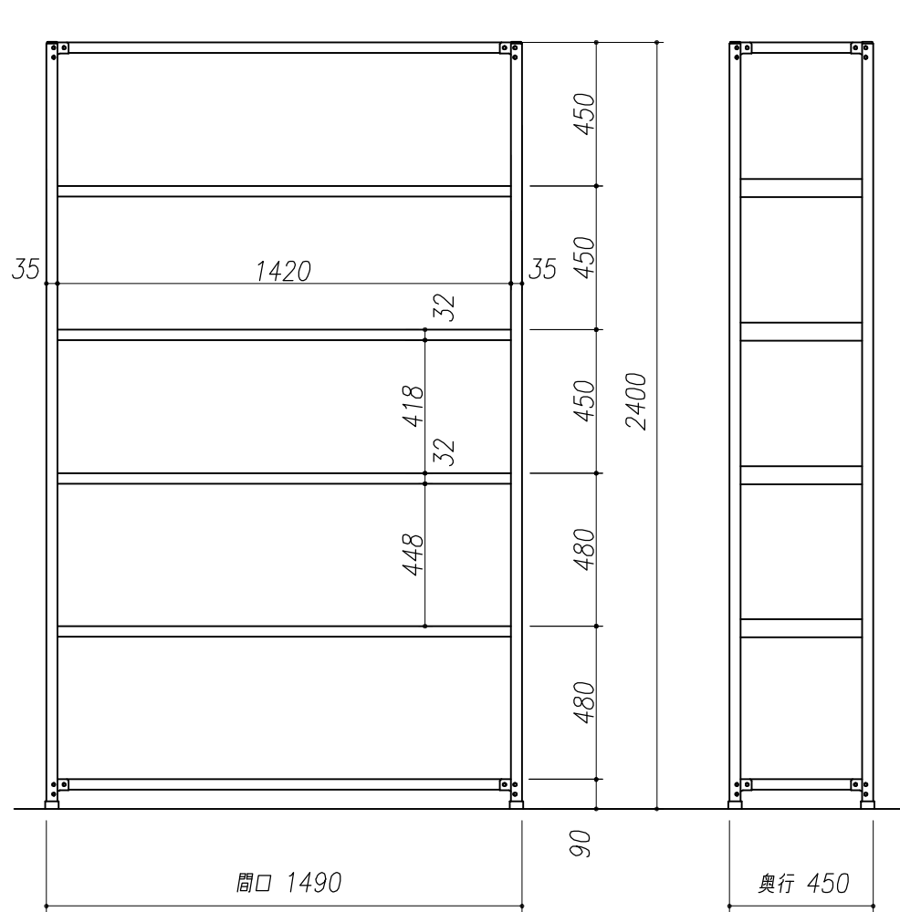
品番：TL85S-16
