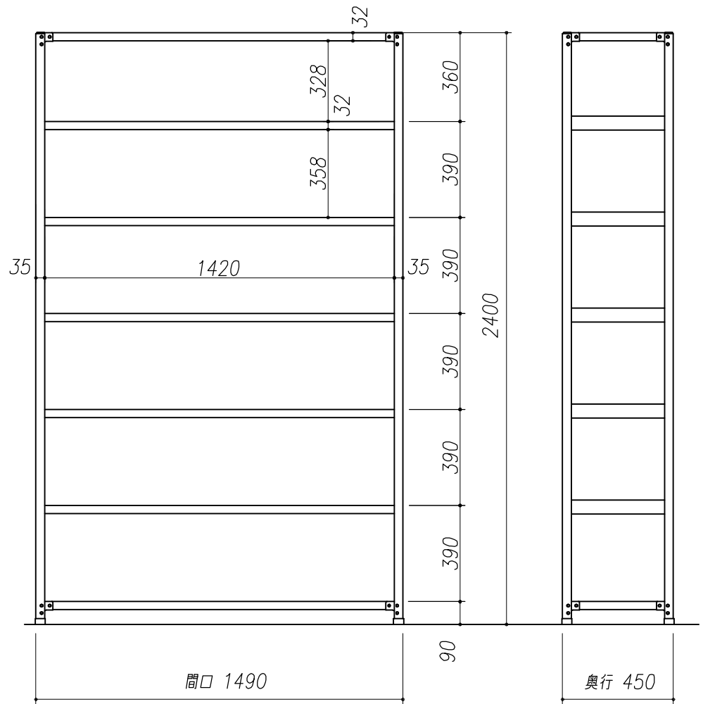
品番：TL85S-17
