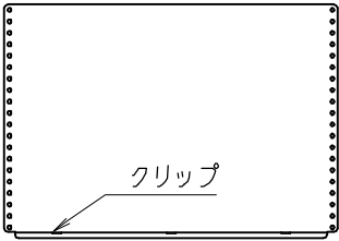
背板 中
