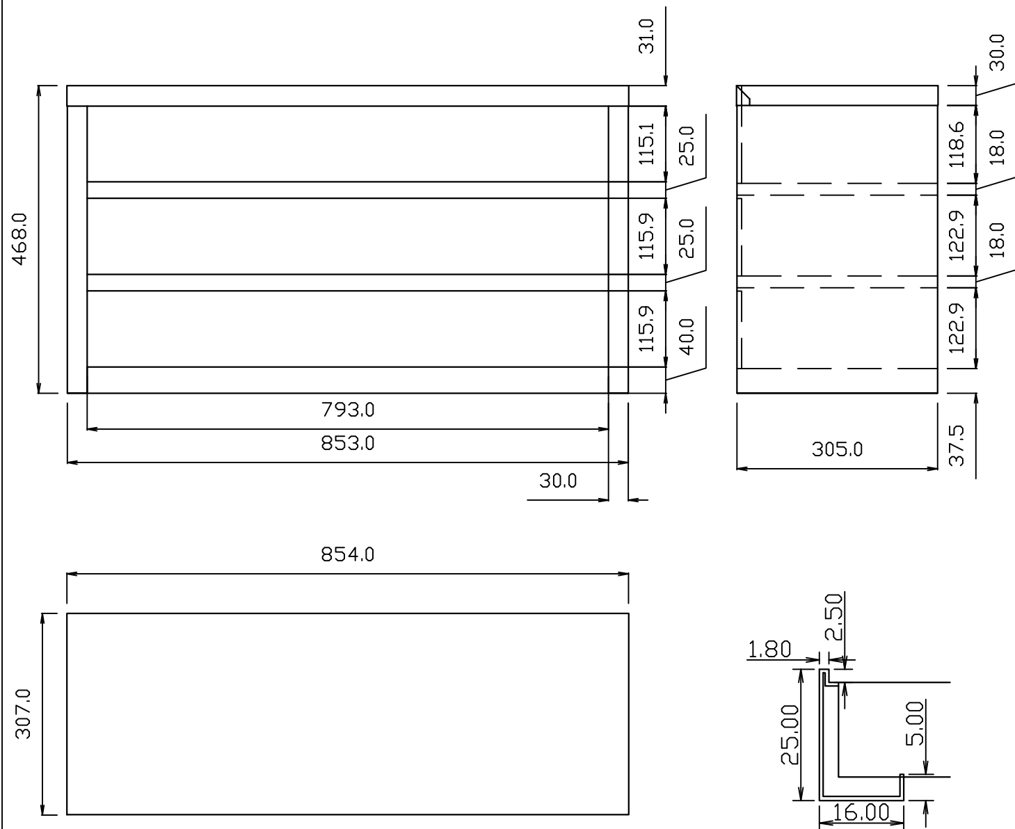
棚板開口部断面拡大図
