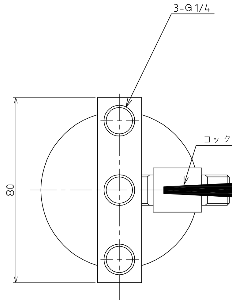
A - A 上面寸法図
