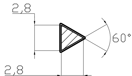
A-A面 拡大
