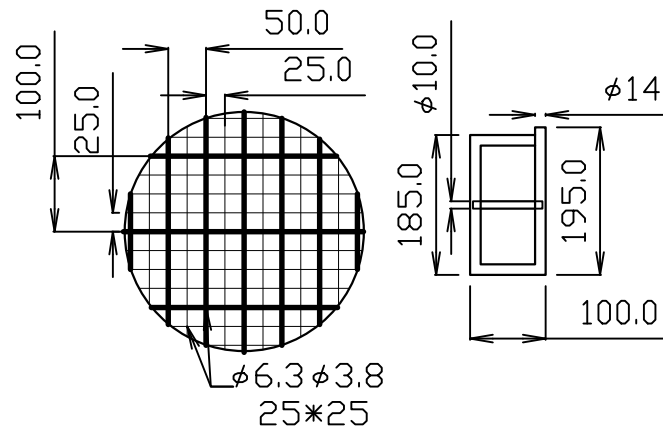
網目寸法 段積み金具
