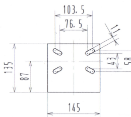
固定車用キャスター板詳細
