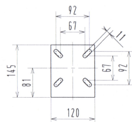
自在車用キャスター板詳細
