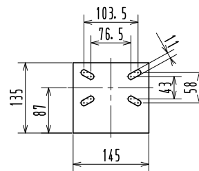
固定車用キャスター板詳細
