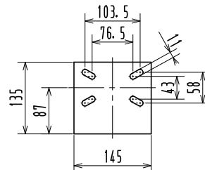
固定車用キャスター板詳細
