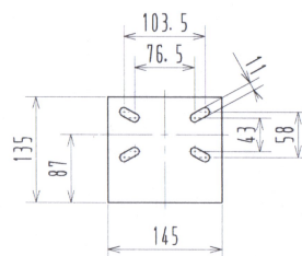
固定車用キャスター板詳細
