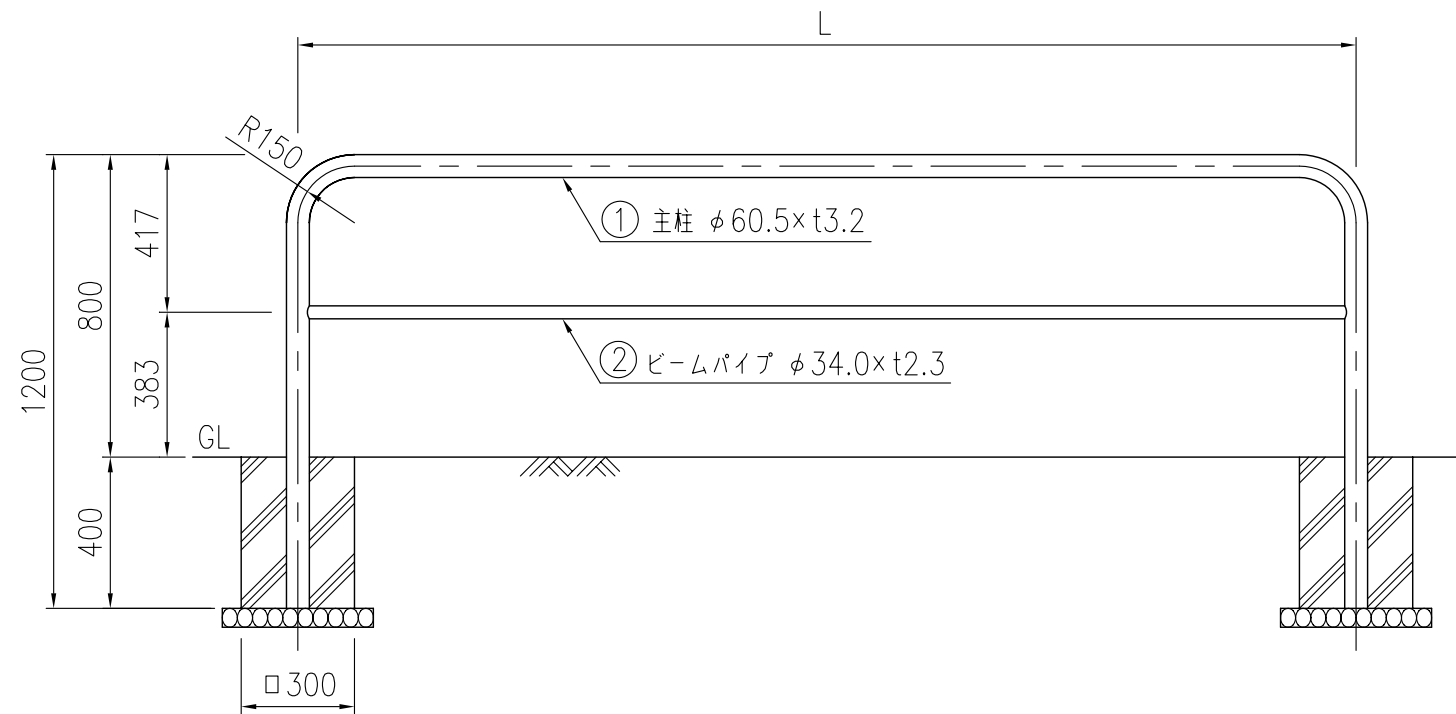
設置図
