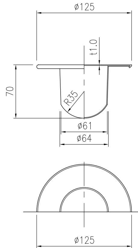
鉄ブタ詳細図
