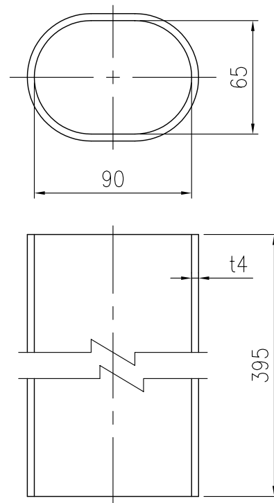
ダ円管詳細図
