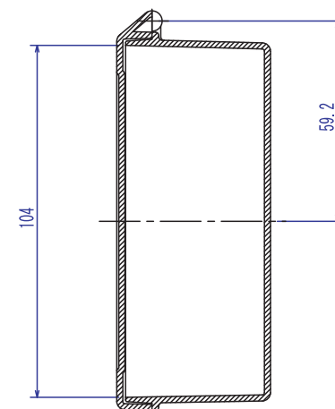
A-A断面図
