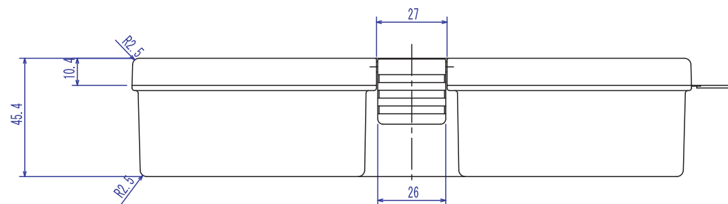
B-B断面図
