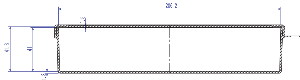
B-B断面図
