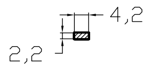
A-A面 拡大
