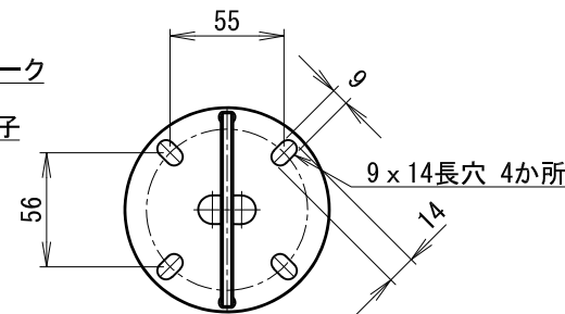
丸座金 拡大図
