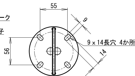
丸座金 拡大図
