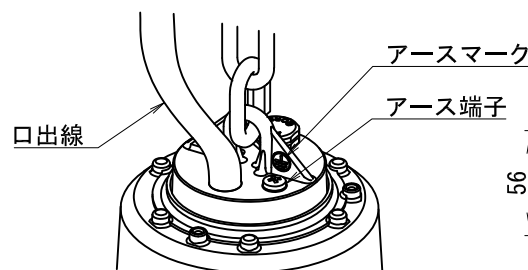
アース接続部 拡大図
