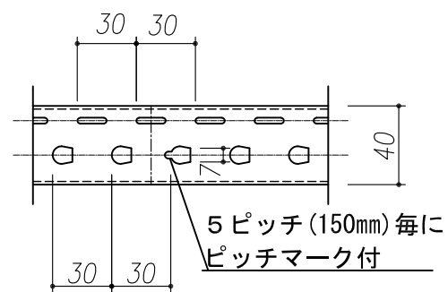
(棚受孔 詳細図)
