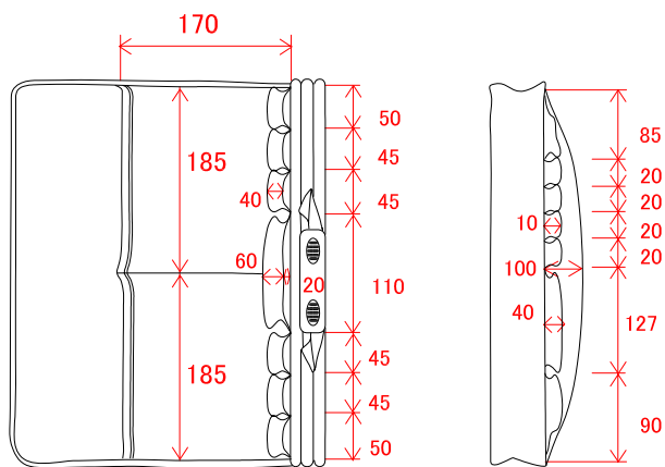
中構造
