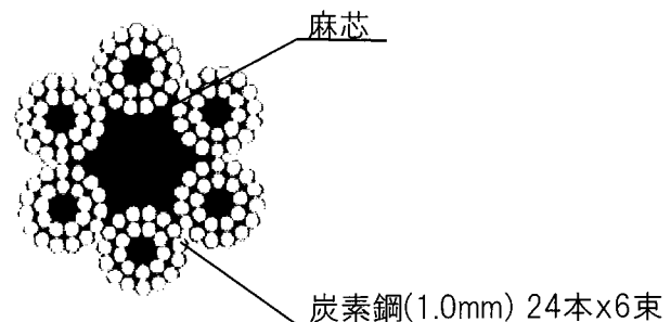
ワイヤロープ断面図
