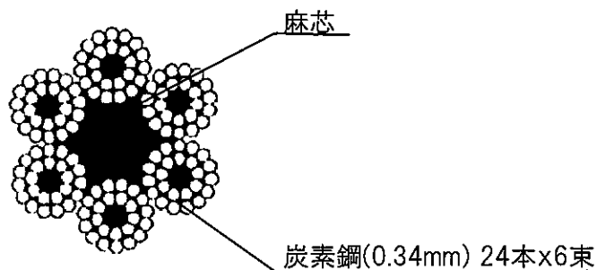
ワイヤロープ断面図
