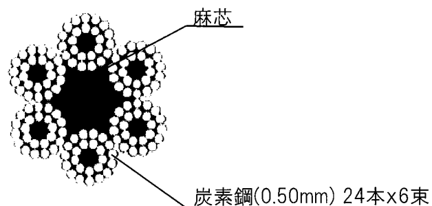
ワイヤロープ断面図
