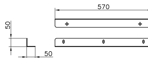
⑪ 転倒防止金具
