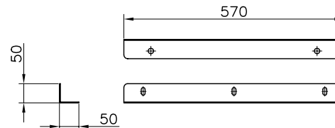
⑩ 転倒防止金具
