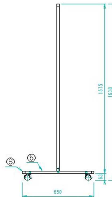
側面図
