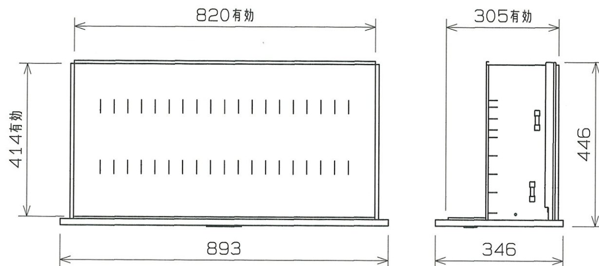
引出詳細図
