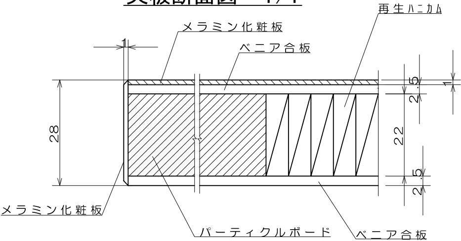
天板断面図 1/1
