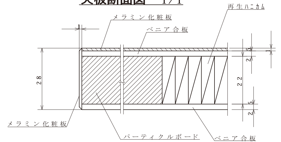
天板断面図 1/1
