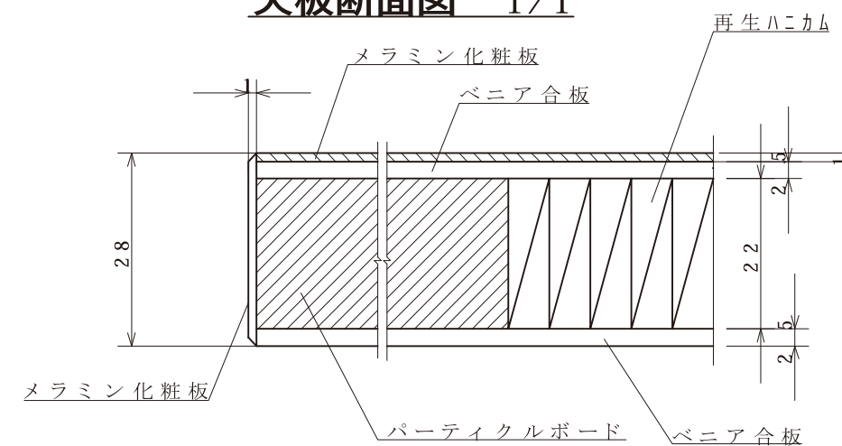
天板断面図 1/1
