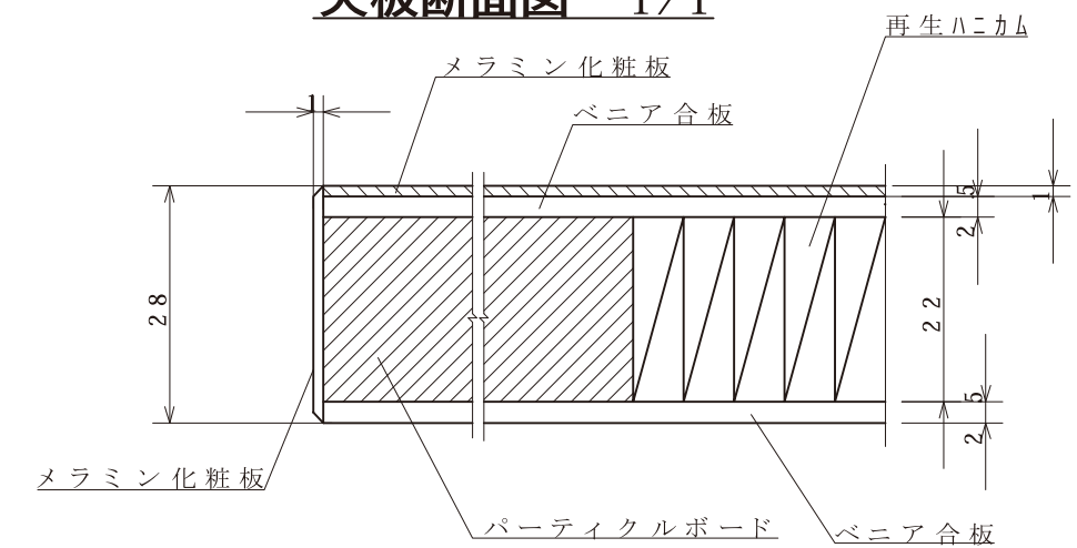
天板断面図 1/1
