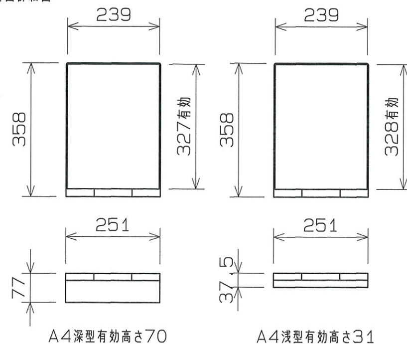
引出詳細図
