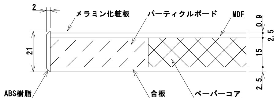
天板断面図 1:6
