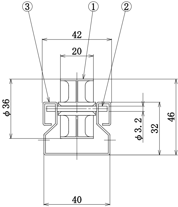
断面詳細
